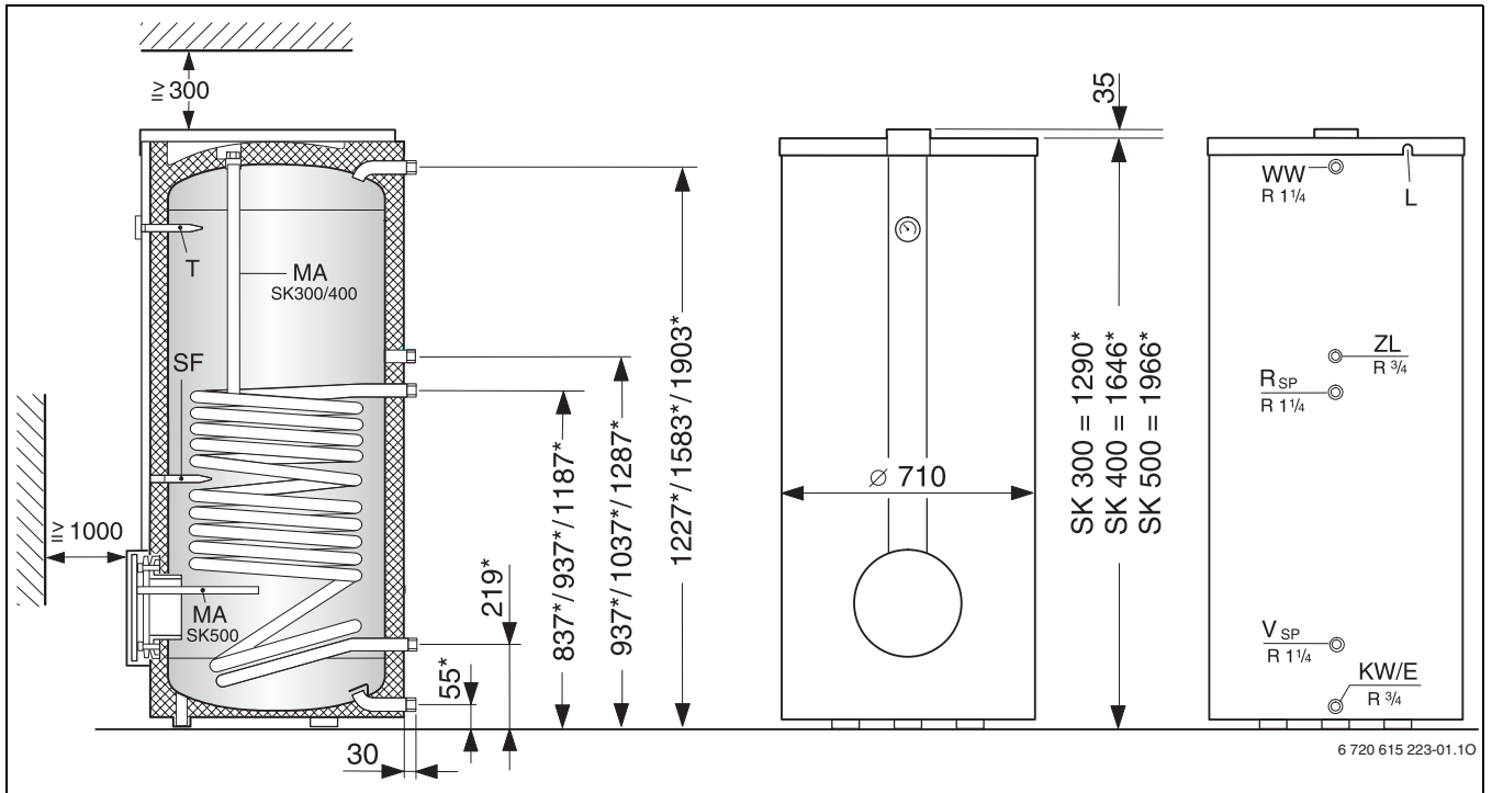
Fig. 1 Dimensiunile menționate în spatele unei linii oblice se raportează la următoarea versiune a boilerului ca mărime.
