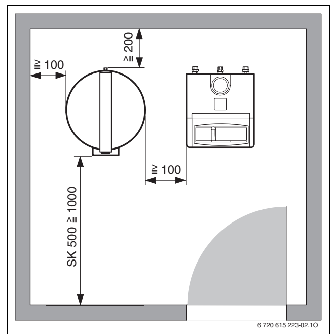
Fig. 2 Distanțe minime recomandate față de perete
