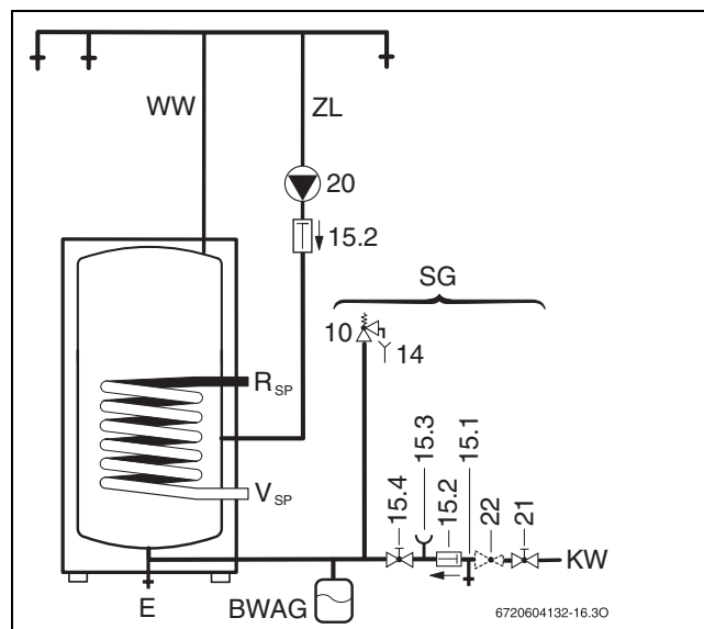
Fig. 6 Schemă de racordare la nivelul apei potabile
